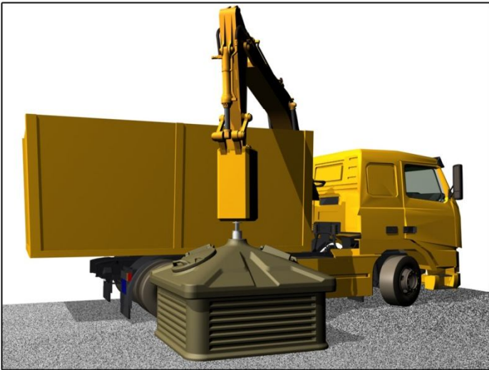
Mise en pace du camion à proximité Saisir le crochet avec la pince
